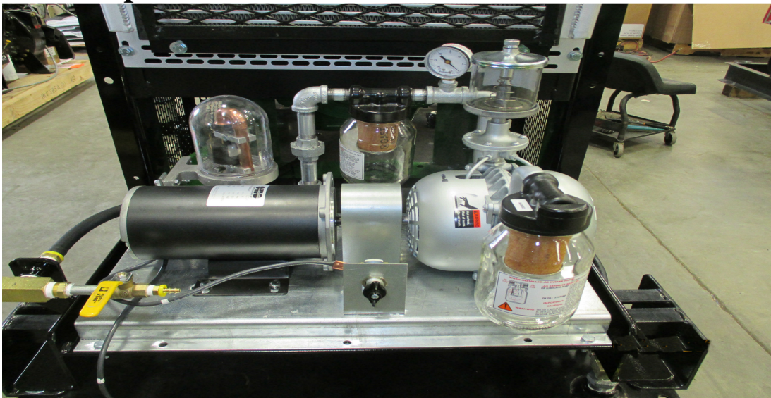
Exhaust primer
